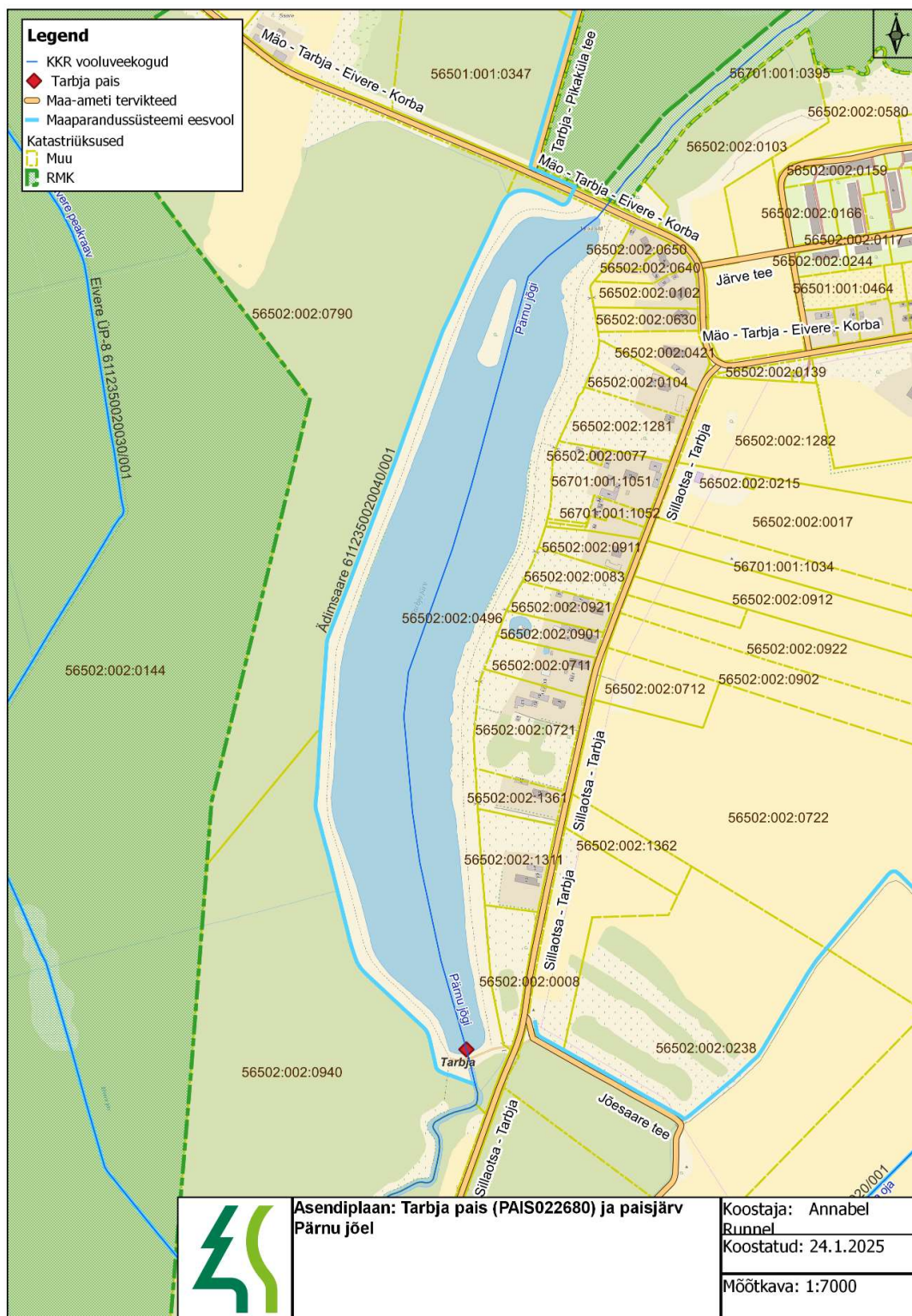
Joonis 1. Tarbja paisu ja paisjärve asendiplaan.
